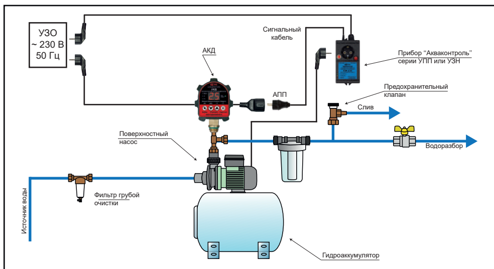
Пример 3. Подключение АКД к УПП или УЗН "Extra Акваконтроль" через адаптер АПП.
