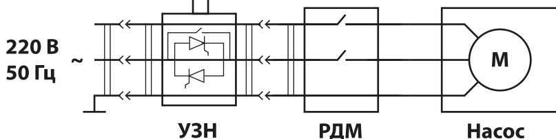
Схема 2. Подключение УЗН после механического реле давления типа РДМ
