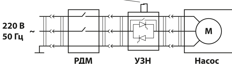
Схема 3. Подключение УЗН к механическому реле давления типа РДМ с помощью управляющего провода
