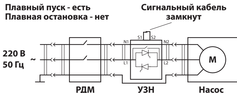
Схема 3. Управление УЗН на DIN рейку с помощью сигнального кабеля
