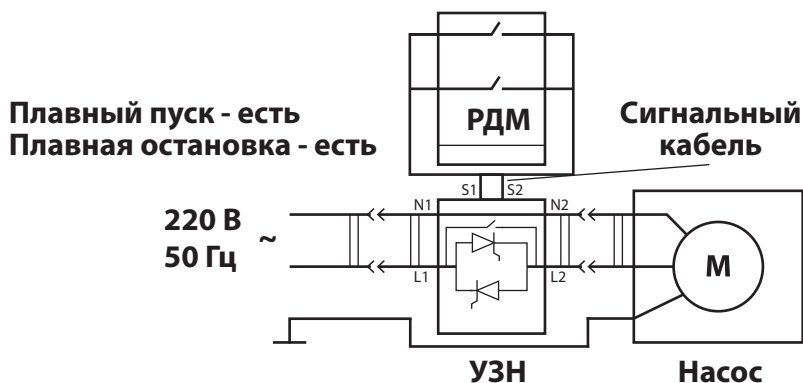
Схема 3. Управление УЗН на DIN рейку с помощью сигнального кабеля
