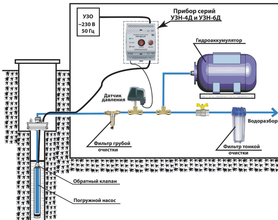
Схема 5. Пример подключения приборов УЗН-4Д и УЗН-6Д “Акваконтроль” с погружным насосом и реле давления типа РД-5/(РДМ).
