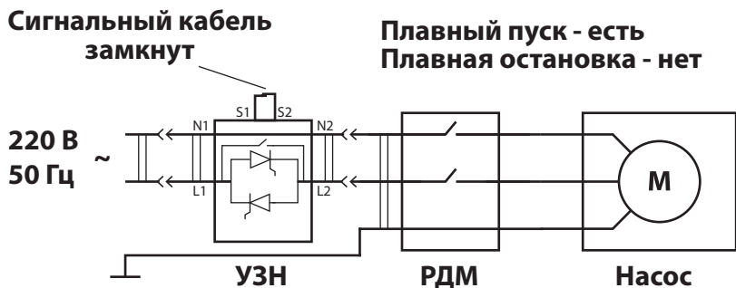
Схема 2. Подключение УЗН на DIN рейку после механического реле давления типа РДМ
