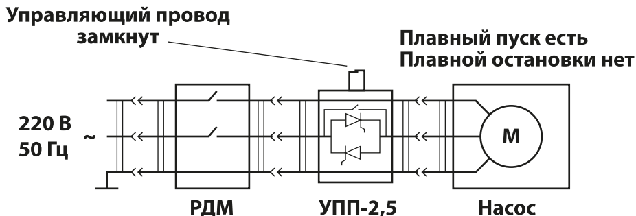
Схема 3. Подключение УПП-2,5 после механического реле давления типа РДМ
